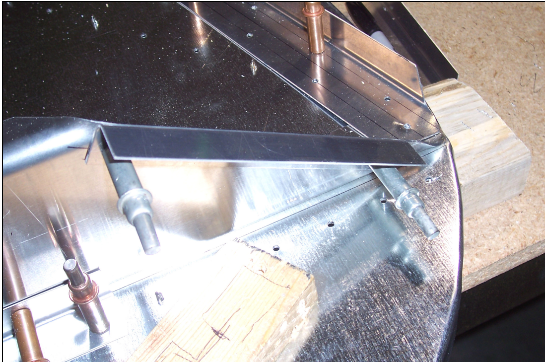
P/N: 6B7-3 Side Brace
