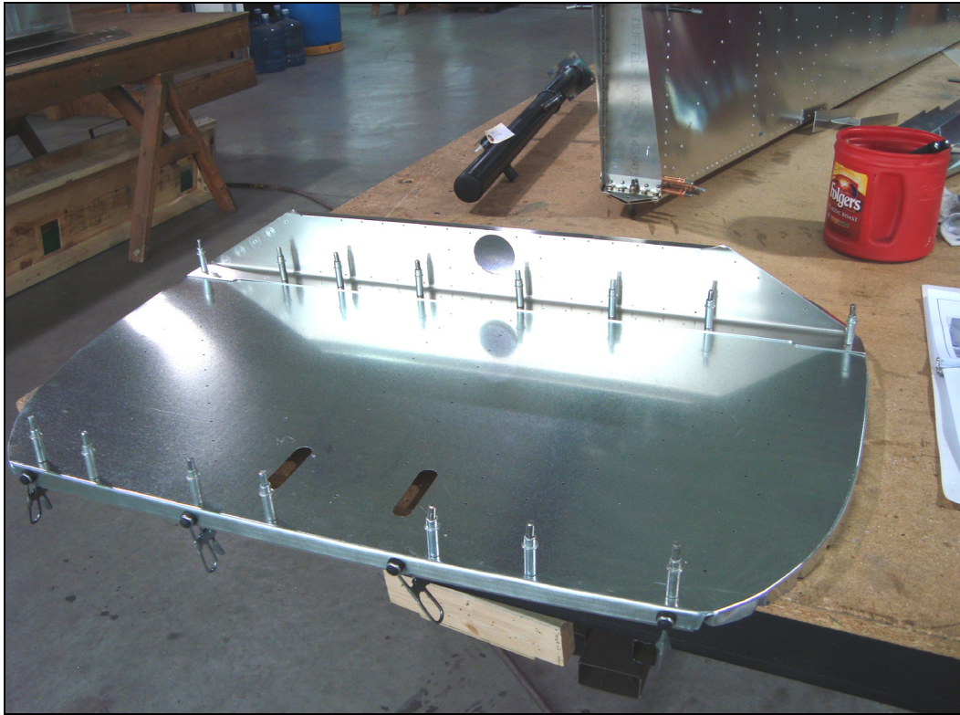
P/N: 6B7-1 Firewall Top Stiffener
