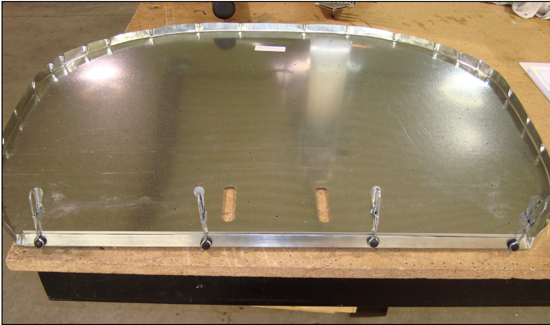
P/N: 6B6-2 Firewall
